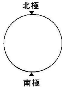
地球の断面図
