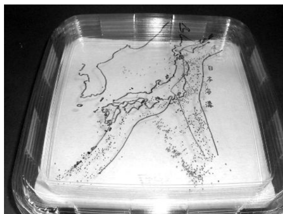
図1 作成した震源立体模型
